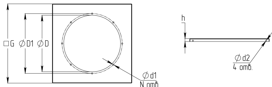
Внешний вид типоразмеров 630-1250
