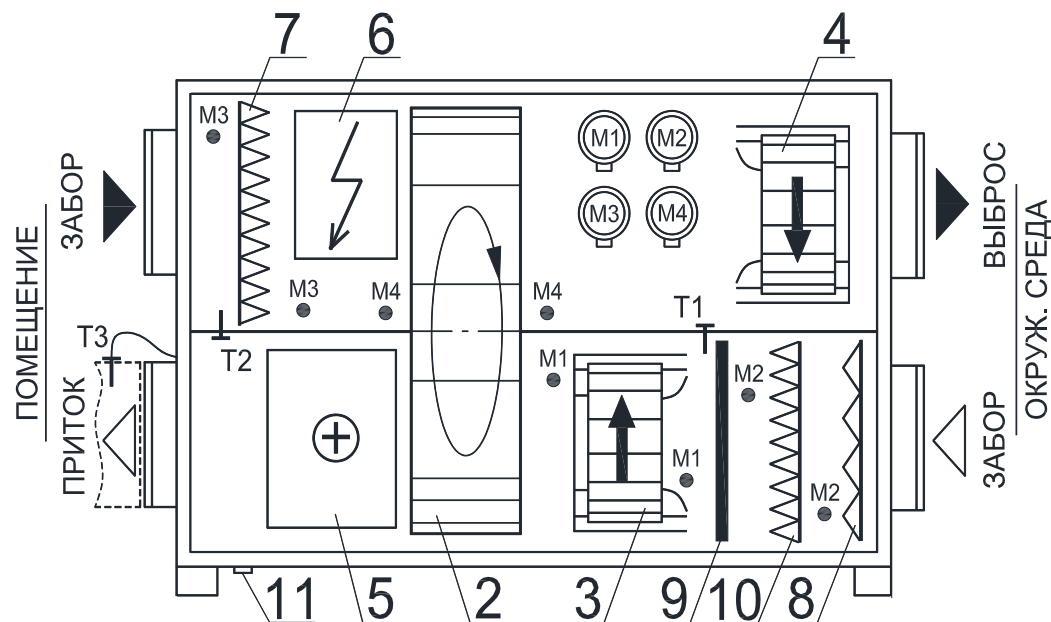
Рисунок 1. Схема компоновки установки на базе роторного регенератора (исполнение - RG, левое - L)
