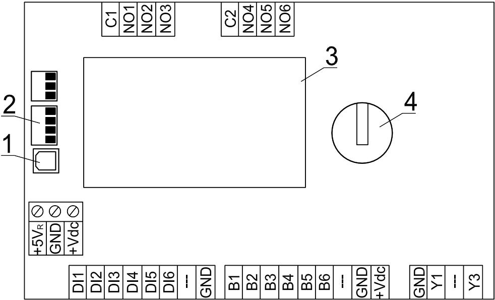
Рисунок 3. Основные элементы конструкции платы контроллера
