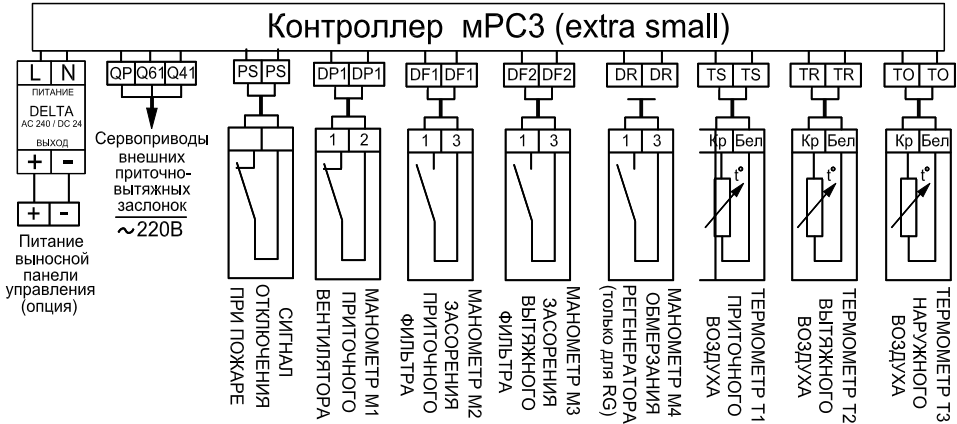
Схема 1. Внешние подключения элементов автоматики к блоку управления
