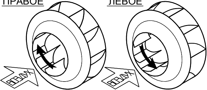
НАПРАВЛЕНИЕ ВРАЩЕНИЯ РАБОЧЕГО КОЛЕСА ПРАВОЕ ЛЕВОЕ
