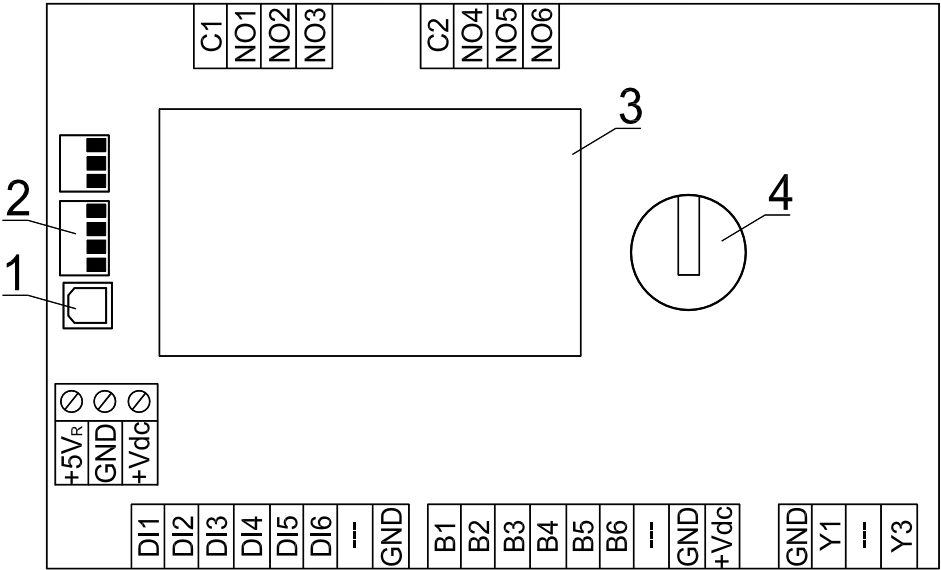
Схема 2. Основные элементы конструкции платы контроллера
